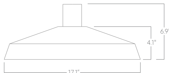
Mars
