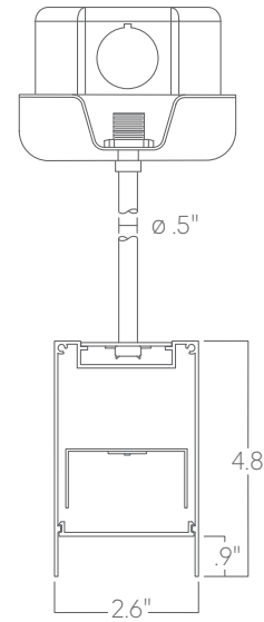
Pendant stem
