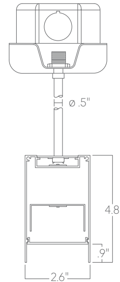
Pendant stem
