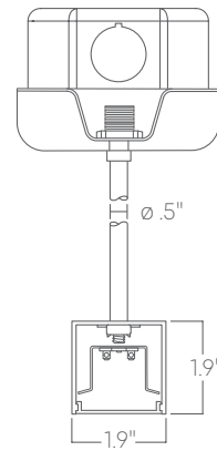
Pendant stem
