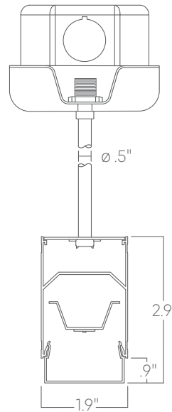
Pendant stem
