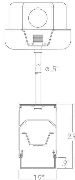
Pendant stem
