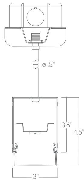
Pendant stem
