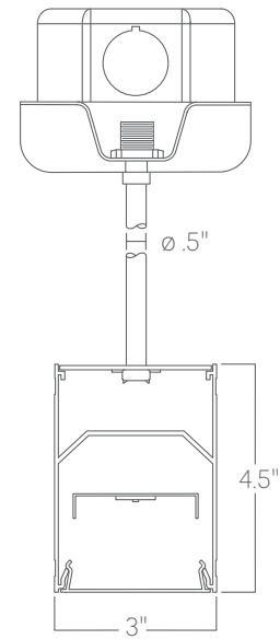
Pendant stem
