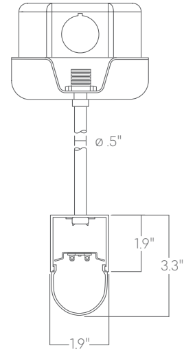
Pendant stem
