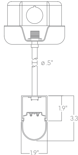
Pendant stem
