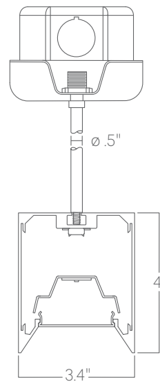
Pendant stem
