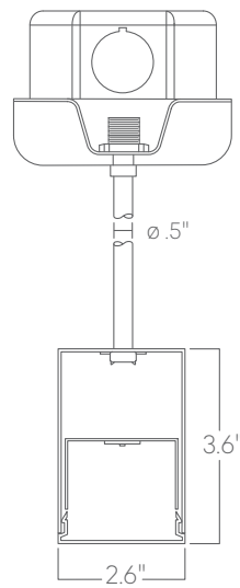
Pendant stem
